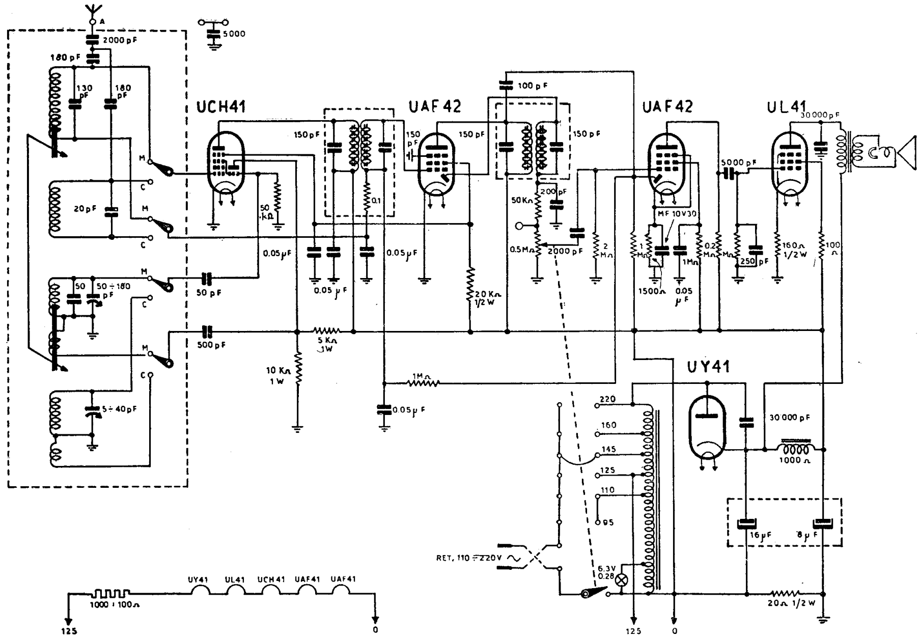
SAVIGLIANO - Mod. 5R - Serie 49/II. Media frequenza 460 kc. Potenza d'uscita 2 watt.
